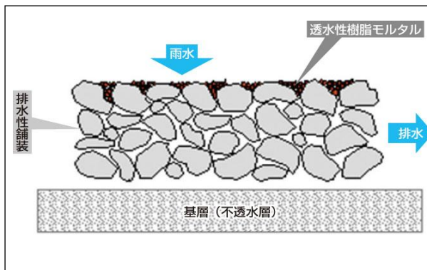
PRMS 舗装の原理
